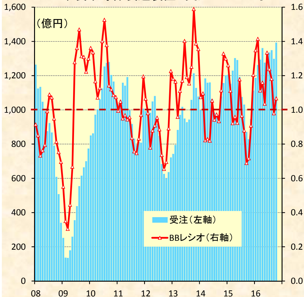
日本製半導体製造装置 受注とBBレシオ
